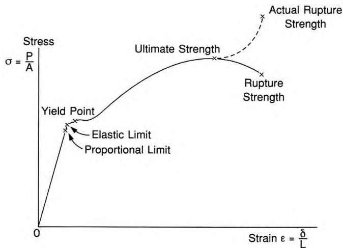
ภาพที่ 2.9 กราฟแสดงความสัมพันธ์ระหว่างความเค้นกับความเครียด
