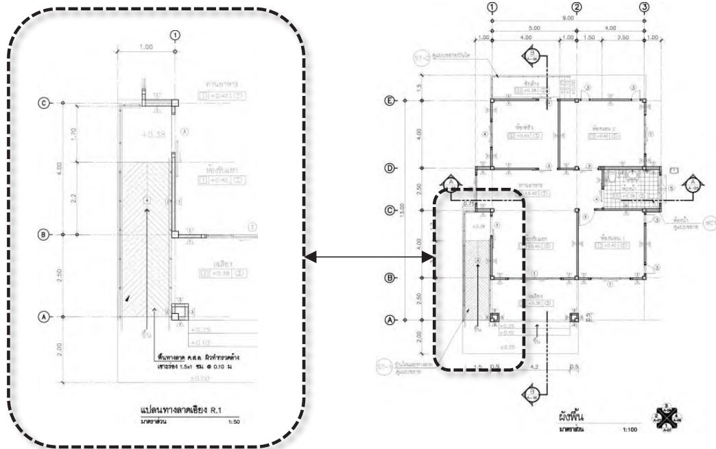
รูปที่ 1.2 ตัวอย่างการจัดวางแบบขยายให้มีทิศทางเดียวกับแบบในแผ่นงาน (ที่มา : ปณิดา มาตรฐาน. 2568)
