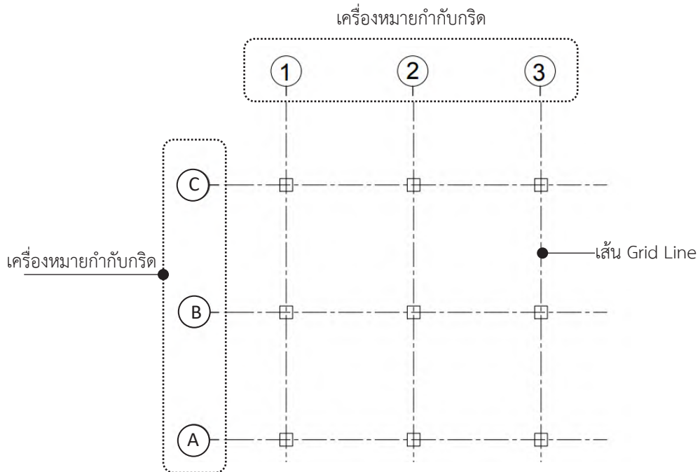
รูปที่ 1.3 ตัวอย่างการเขียนกริดโครงสร้างแสดงแนวศูนย์กลางของเสา (ที่มา : ปกติ มาตนอก. 2568)
