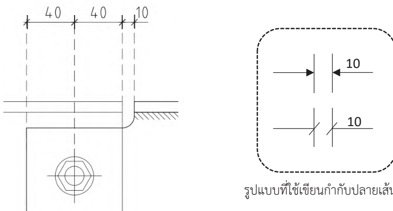
รูปที่ 1.5 ตัวอย่างการเขียนมิติในที่แคบ
