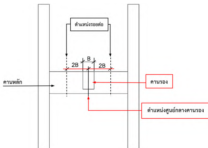
รูปที่ 1.5 การเลื่อนรอยต่อในการหยุดการเทคอนกรีต เมื่อรอยต่อวางตรงกับคานรอง
