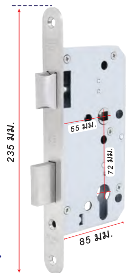
Lock case & Mortise Lockset กล่องกลไกระบบมอร์ติสล็อก
